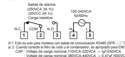
Serie SPR1
